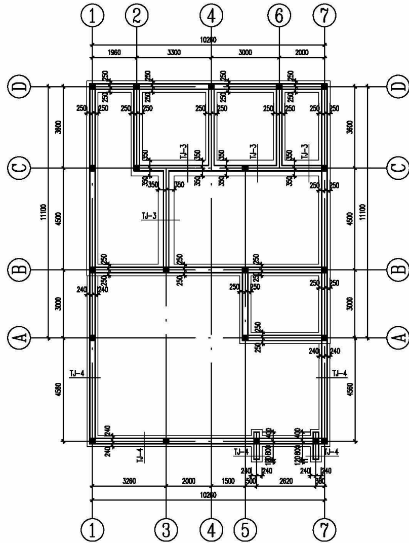
基础平面图
