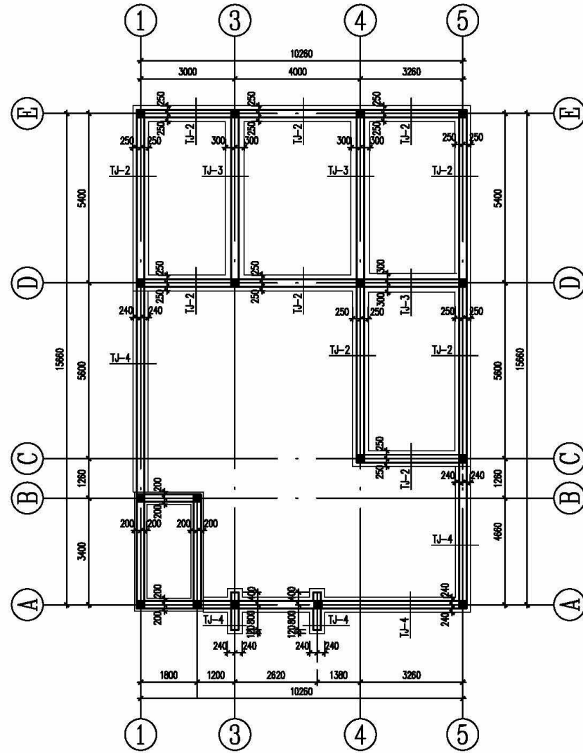
基础平面图
