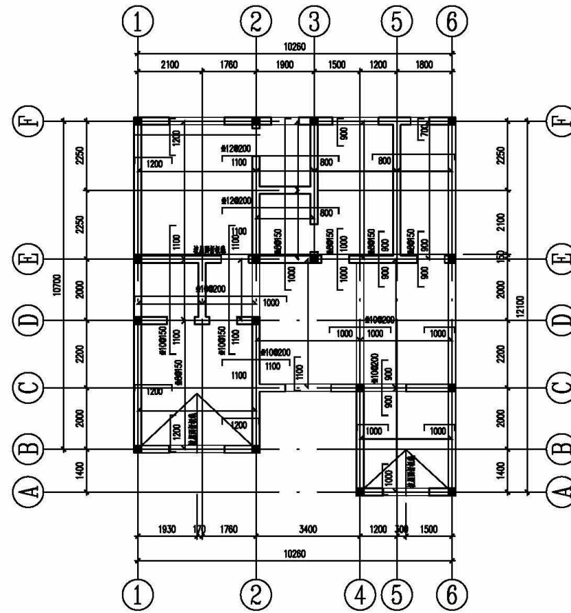
坡屋面配筋图
