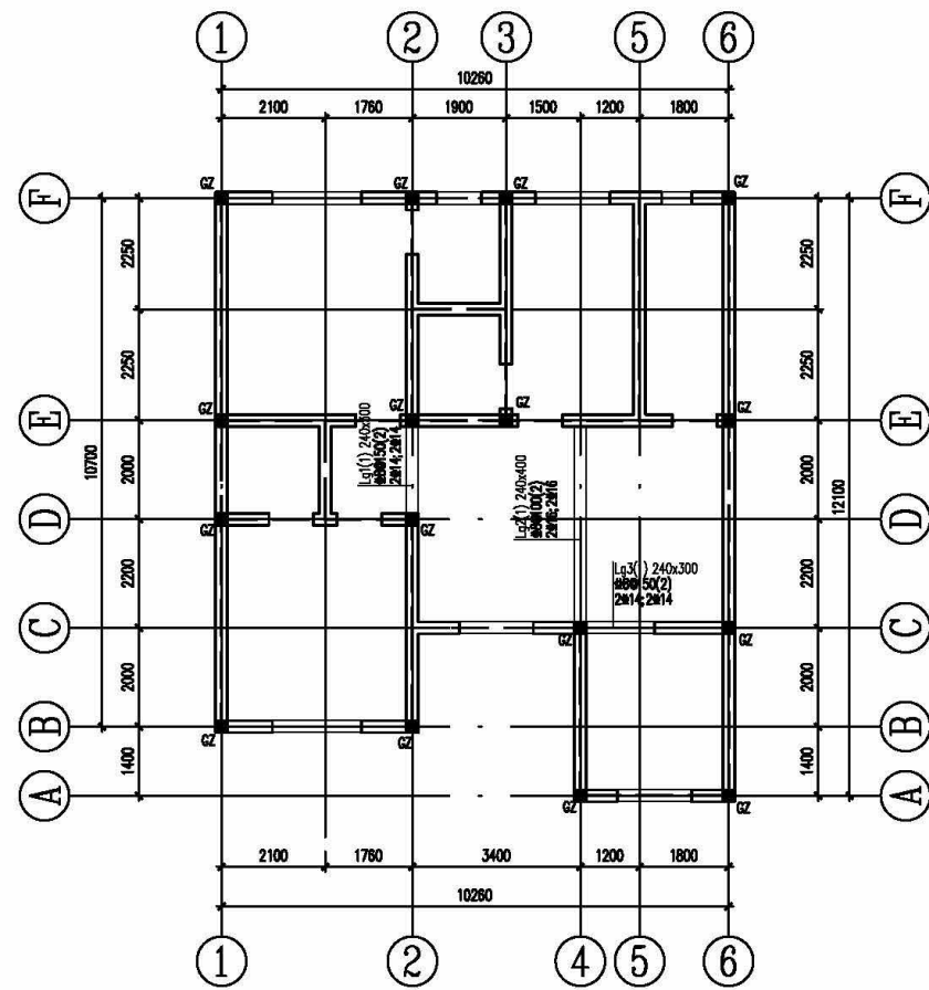
坡屋面结构平面布置图
