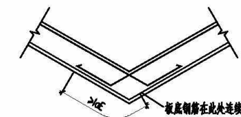
现浇板下折时配筋大样
