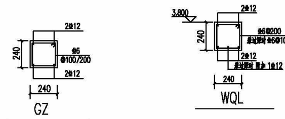
坡屋面配筋图
